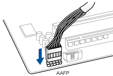
安装前面板音频连接排针
